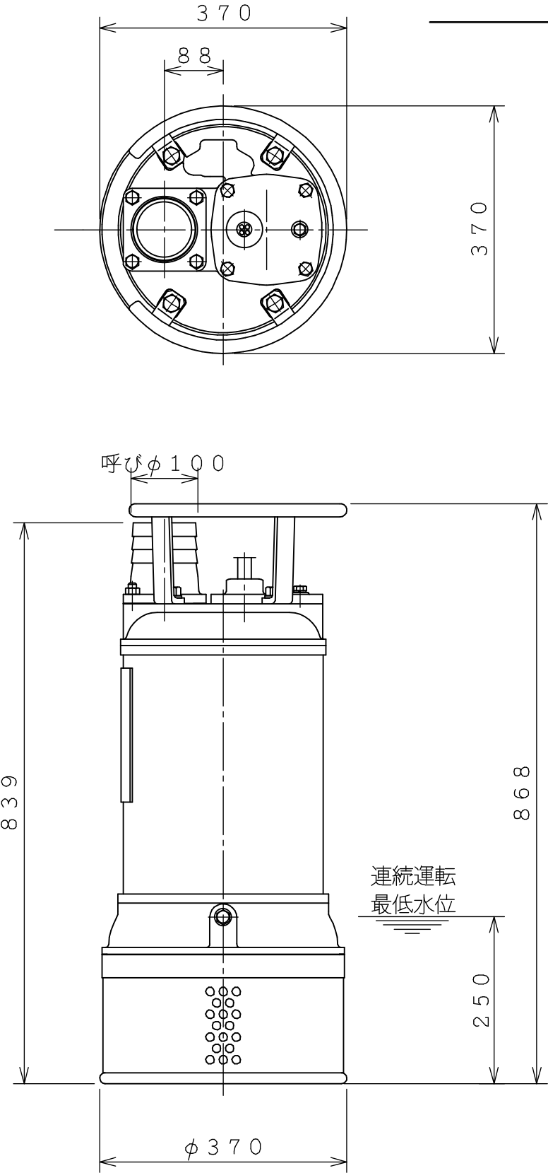
外形寸法図
