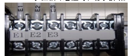
TB2: 水位計(電極等)端子詳細
