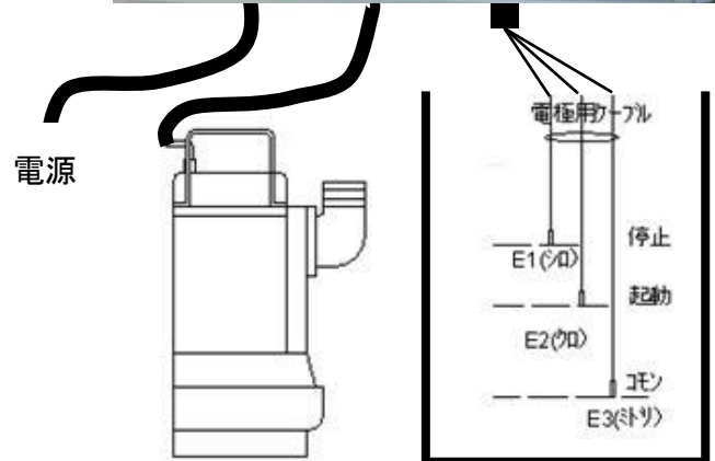
TB1: 電源・ポンプ端子詳細
